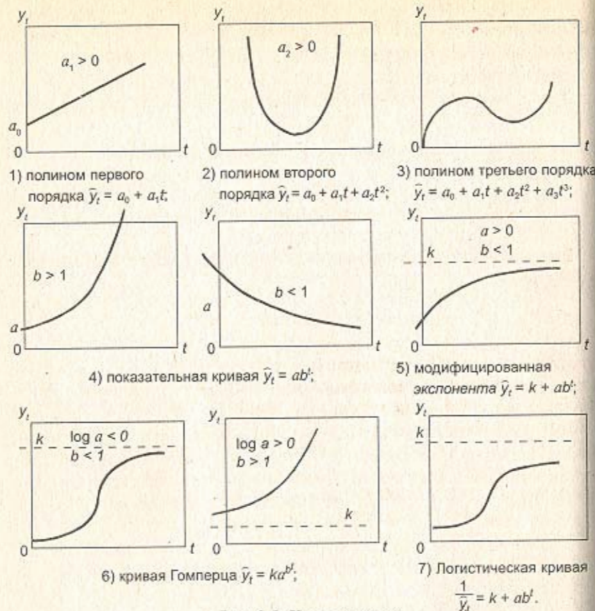
Рис. 3.1. Кривые роста
