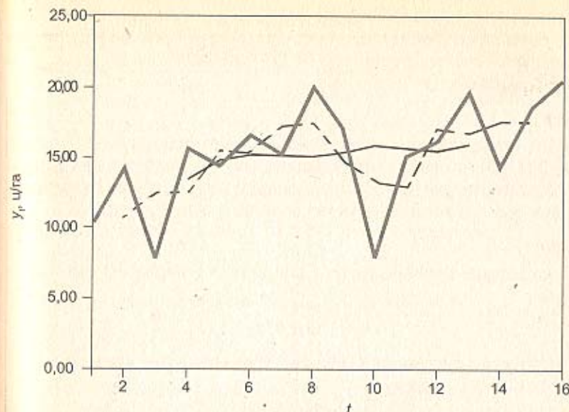
Рис. 2.2. Сглаживание ряда урожайности с помощью скользящих средних:
