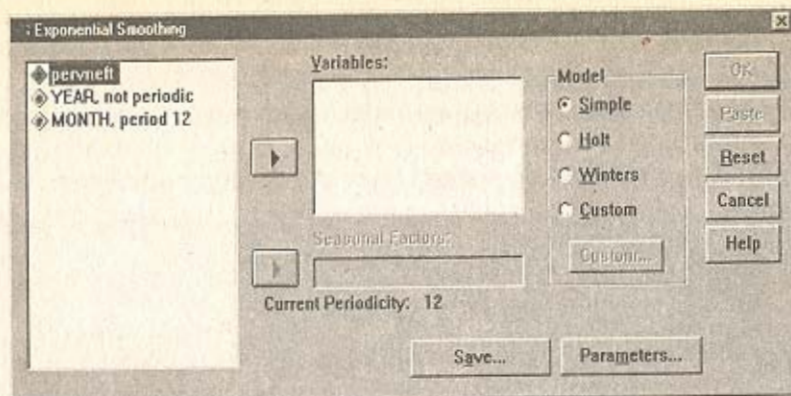
Рис. 7.4. Вид окна «Экспоненциальное сглаживание» (Exponential Smoothing)
