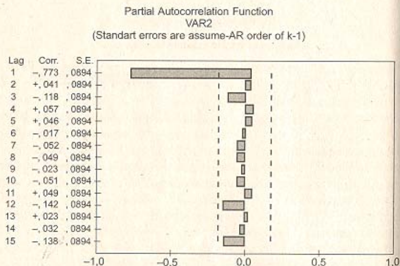
Рис. 6.4. ЧАКФ для ряда, генерированного моделью AR(1) y_t = -0,8y_{t-1} + \varepsilon_t
