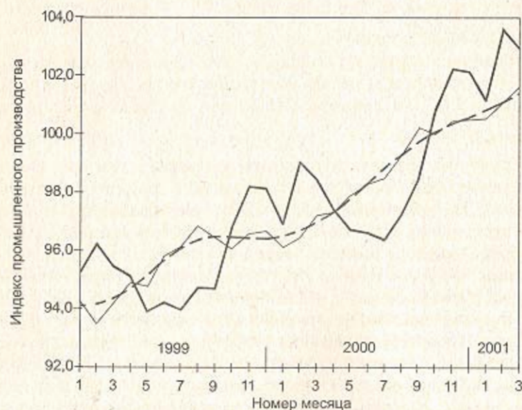
Рис. 4.2. Сезонная корректировка индекса промышленного производства в топливной промышленности (% к декабрю 1997 г.): — с исключением календарного фактора; - - - с исключением сезонной компоненты; — — — тренд
