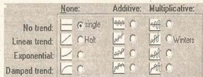
Рис. 5.4. Фрагмент меню в ППП STATISTICA: адаптивные модели, основанные на процедуре экспоненциального сглаживания
