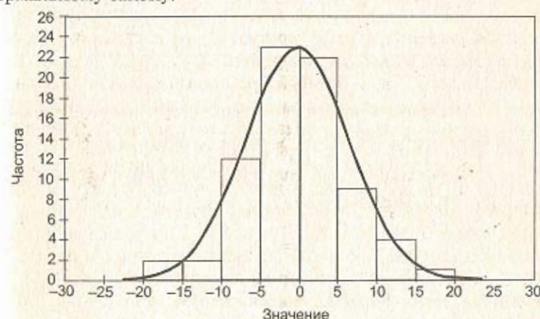
Рис. 3.3. Гистограмма остатков:
