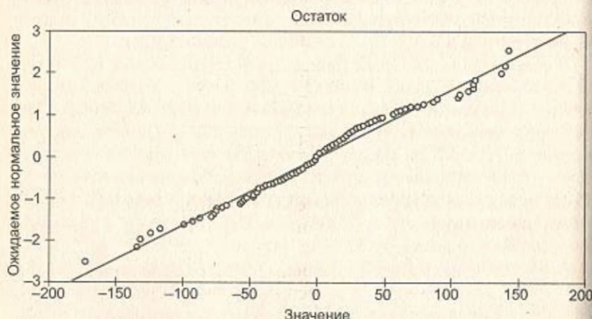
Рис. 3.4. График остатков на нормальной вероятностной бумаге
