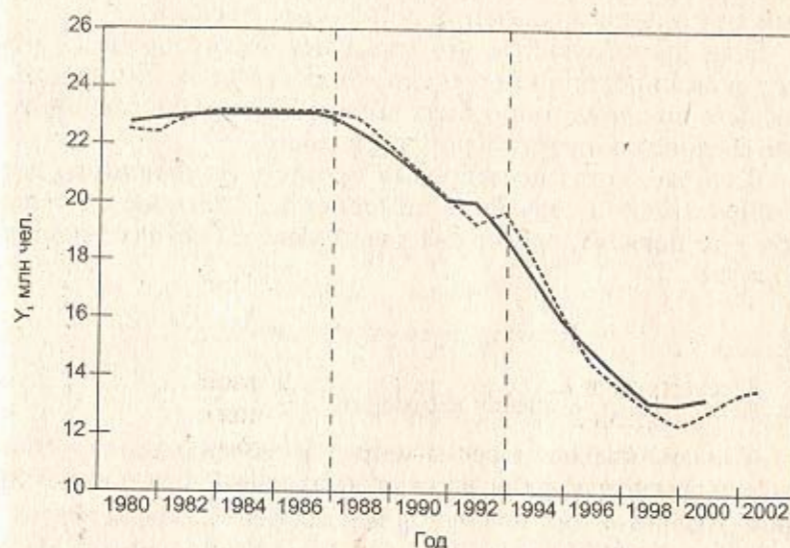
Рис. 5.3. Прогнозирование среднегодовой численности Y промышленно-производственного персонала с помощью модели Ч. Хольта
