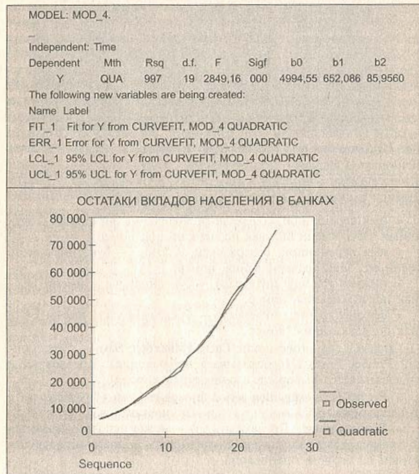
Рис 7.3. Результаты оценивания модели кривой роста с помощью процедуры Curve Estimation
