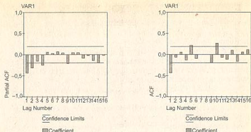
Рис. 7.15. Графики АКФ (ACF) и ЧАКФ (PACF)
