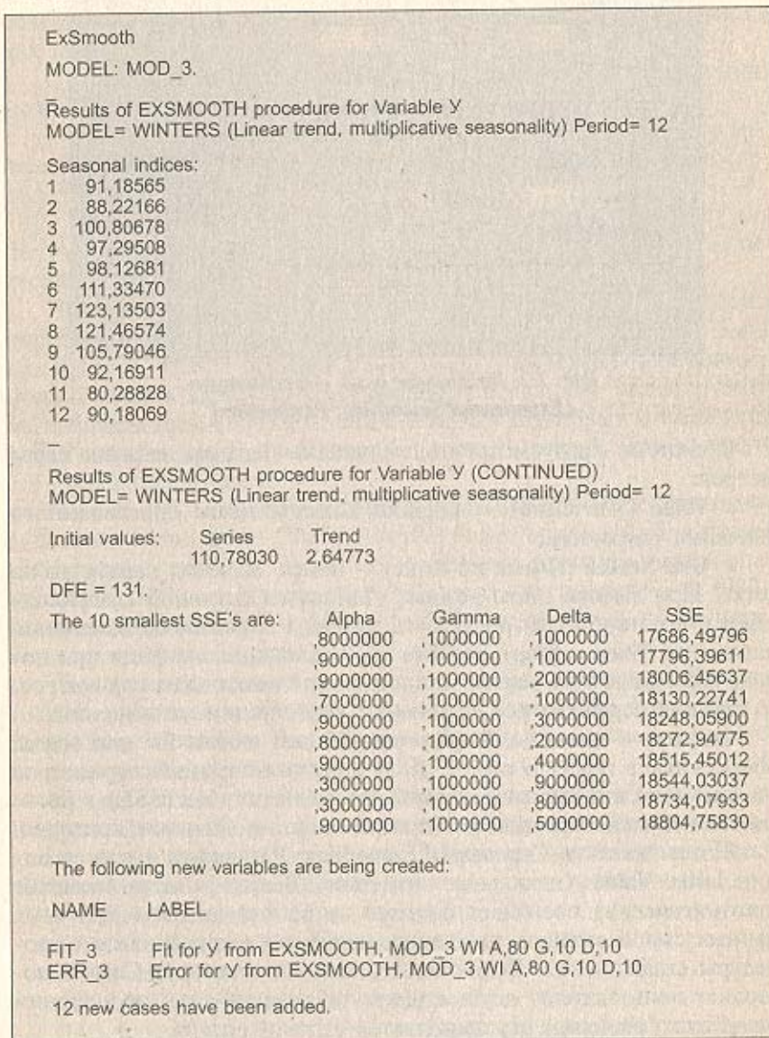
Рис. 7.8. Вариант отчета экспоненциального сглаживания (линейный тренд, мультипликативная сезонность), полученного в SPSS — Viewer
