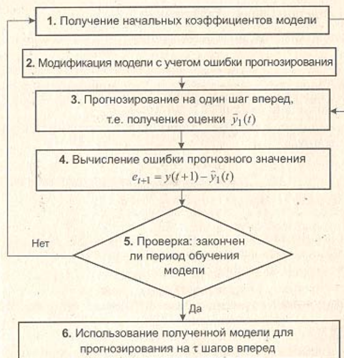
Рис. 5.1. Схема построения адаптивных моделей прогнозирования: y(t) — фактические уровни временного ряда; \hat{y}_t(t) — прогноз, сделанный в момент t на t единиц времени (шагов) вперед; e_{t+1} — ошибка прогноза, полученная как разница между фактическим и прогнозным значением показателя в точке (t+1)
