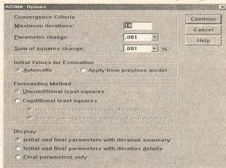
Рис. 7.12. Вид диалогового окна ARIMA: Options
