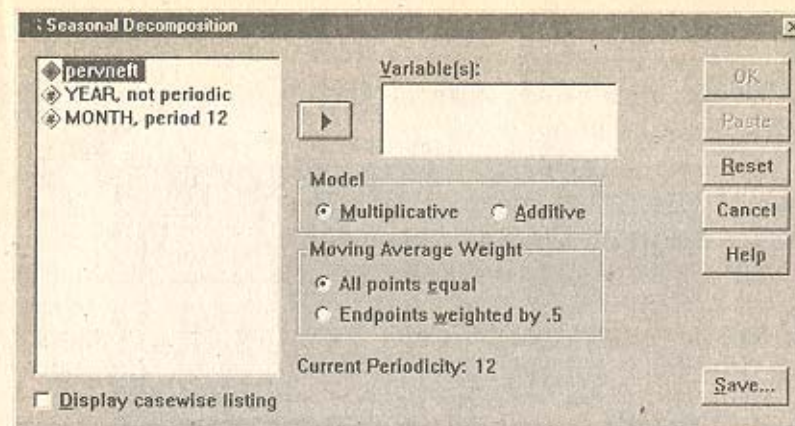
Рис. 7.16. Вид диалогового окна «Сезонная декомпозиция» (Seasonal Decomposition)
