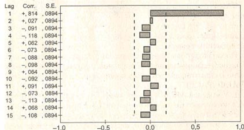
Рис. 6.2. ЧАКФ для ряда, генерированного моделью AR(1) y_t = 0,8y_{t-1} + \varepsilon_t
