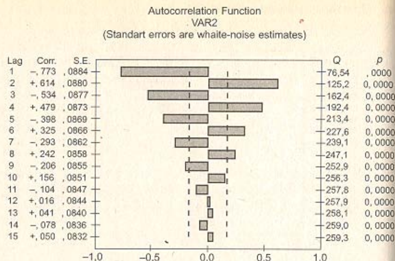
Рис. 6.3. АКФ для ряда, генерированного моделью AR(1) y_t = -0,8y_{t-1} + \varepsilon_t . Корень -1,25
