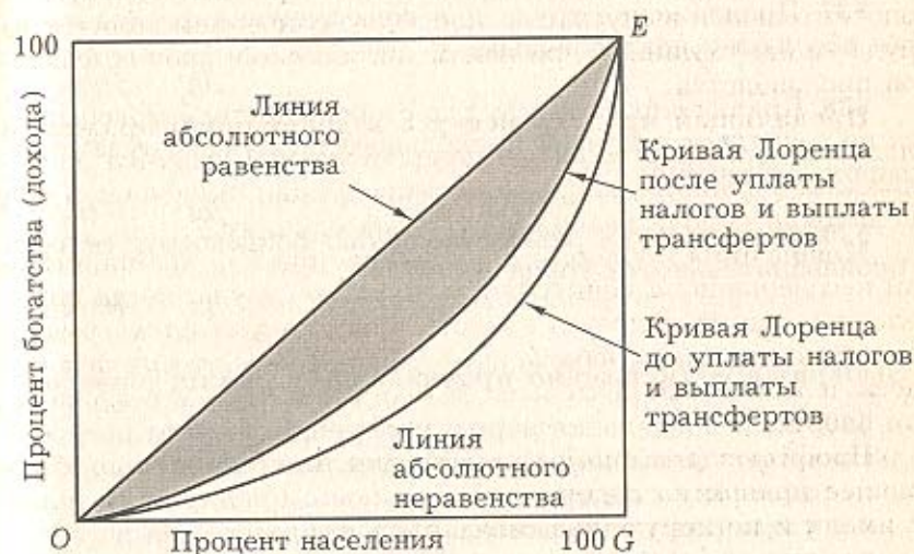
Рис. 9.1. Кривая Лоренца
