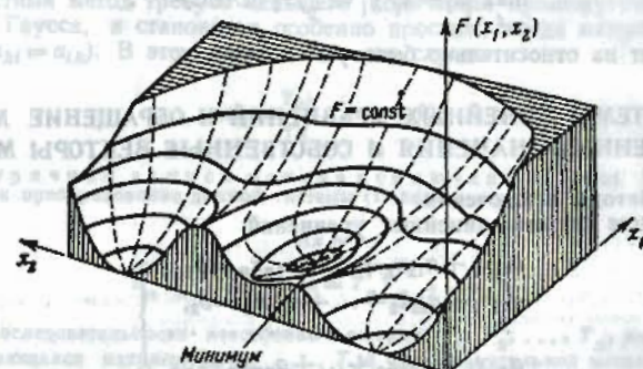
Рис. 20.2-1. График исследуемой на минимум функции в случае двух независимых переменных. Показано три минимума, линии уровня и линия наискорейшего спуска. В этом примере все три минимума функции F(x_1, x_2) имеют одно и то же нулевое значение.
