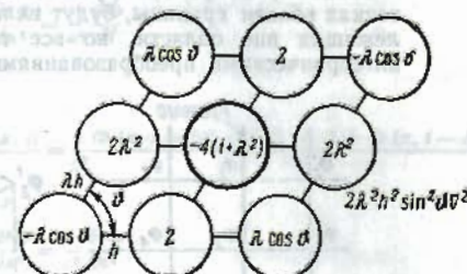
Рис. 20.9-4. Центрально-разностный оператор, применяемый для косоугольной сетки декартовых координат. Относительная погрешность имеет порядок h^2 .
