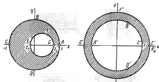
Рис. 14. w = \frac{z-a}{az-1} ; a = \frac{1+x_1x_2 + \sqrt{(1-x_1^2)(1-x_2^2)}}{x_1+x_2} ; R_0 = \frac{1-x_1x_2 + \sqrt{(1-x_1^2)(1-x_2^2)}}{x_1-x_2} (\omega > 1 \text{ в } R_0 > 1, \text{ если } -1 < x_2 < x_1 < 1)
