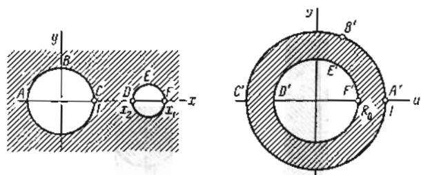
Рис. 15. w = \frac{z-a}{az-1} ; a = \frac{1+x_1x_2 + \sqrt{(x_1^2-1)(x_2^2-1)}}{x_1+x_2} ; R_0 = \frac{x_1x_2-1 + \sqrt{(x_1^2-1)(x_2^2-1)}}{x_1-x_2} (x_2 < a < x_1 \text{ и } 0 < R_0 < 1, \text{ если } 1 < x_2 < x_1)
