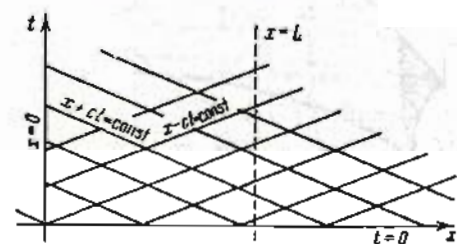
Рис. 10.3-2. Характеристика для одномерного волнового уравнения \frac{\partial^2 \Phi}{\partial x^2} - \frac{1}{c^2} \frac{\partial^2 \Phi}{\partial t^2} = 0 .
