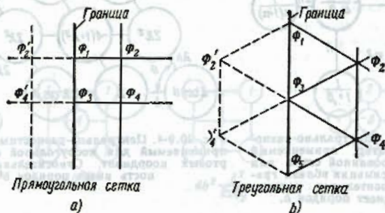
Рис. 20.9-7. Представление краевых условий для \nabla^2 \Phi = 0 или \nabla^4 \Phi = 0 . Сетка продолжена влево от данной границы и введены «отраженные значения» \Phi'_2 = \Phi_2 , \Phi'_4 = \Phi_4 для представления условия \partial\Phi/\partial n = 0 на границе разностным отношением. Краевое условие \Phi = 0 , \nabla^2 \Phi = 0 (например, свободный край упругой пластины) представляется подобным же образом через \Phi_1 = \Phi_3 = 0 , \Phi'_2 = -\Phi_2 , \Phi'_4 = -\Phi_4 .
