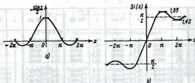
Рис. 21.3-1. Графики функций \frac{\sin x}{x} и \operatorname{Si}(x) .
