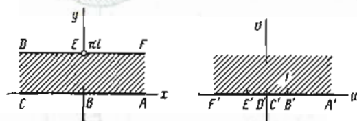
Рис. 6. w = e^z .
