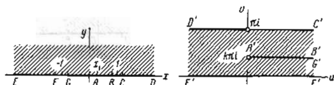
Рис. 22. w = k \ln \frac{z - x_1}{1 - k} + \ln 2(1 - k) + \pi i - k \ln(z + 1) - (1 - k) \ln(z - 1); x_1 = 2k - 1.
