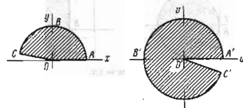
Рис. 1. w = z^2
