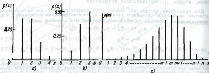
Рис. 18.8-1. Биномиальное распределение:
