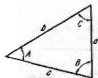
Рис. 1.11-2. Косугольный треугольник.
