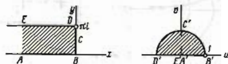
Рис. 7. w = e^z .
