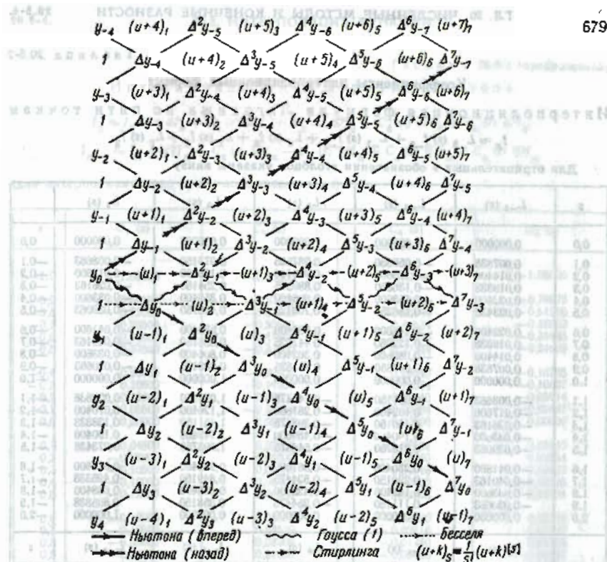
Рис. 20.5-1. Ромбовидная диаграмма для интерполяционных формул. Сокращенное обозначение
