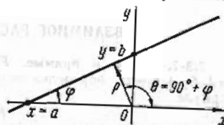
Рис. 2.2-1. Уравнение прямой.
