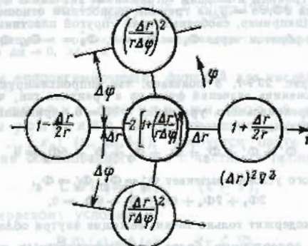
Рис. 20.9-5. Центрально-разностный оператор, применяемый для сетки полярных координат r, \varphi . Относительная погрешность имеет порядок r \Delta r \Delta \varphi . Удобна сетка, градуированная соотношением \Delta r = r \Delta \varphi .
