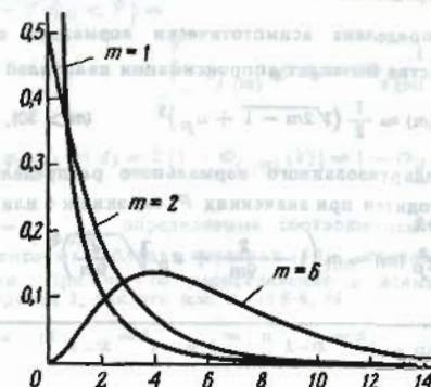
Рис. 19.5-1. \chi^2 -распределение для различных значений m .
