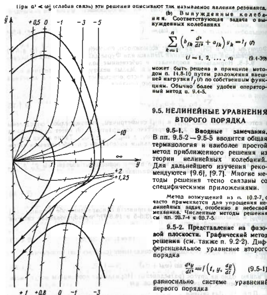
Рис. 9.5-1. Изоклины, направления поля и некоторые решения дифференциального уравнения
