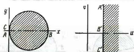
Рис. 5. w = 1/z .
