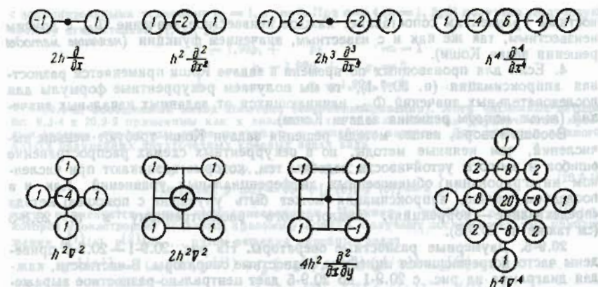
Рис. 20.9-1. Операторы для центрально-разностной аппроксимации (прямоугольная сетка декартовых координат; \Delta x = \Delta y = h ). Относительная погрешность имеет порядок h^2 .
