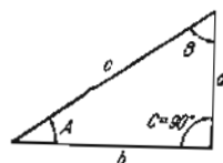
Рис. 1.11-1. Прямоугольный треугольник.
