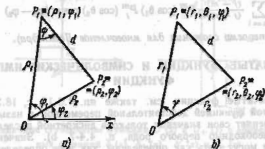
Рис. 21.8-9. Геометрическая иллюстрация к теореме сложения.
