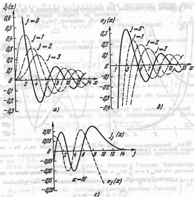
Рис. 21.8-6. Сферические функции Бесселя.
