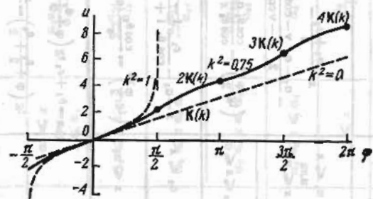
Рис. 21.6-2. Неполный эллиптический интеграл первого рода F(\varphi, k) как функция от \varphi , для трех разных значений k .
