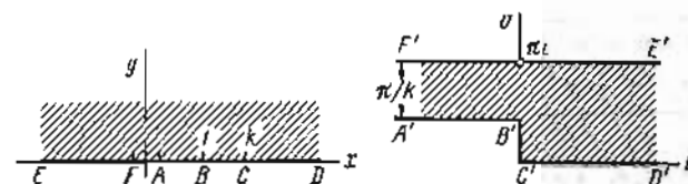
Рис. 30. w = \operatorname{Arch} \left( \frac{2z - k - 1}{k - 1} \right) - \frac{1}{k} \operatorname{Arch} \left[ \frac{(k + 1)z - 2k}{(k - 1)z} \right]
