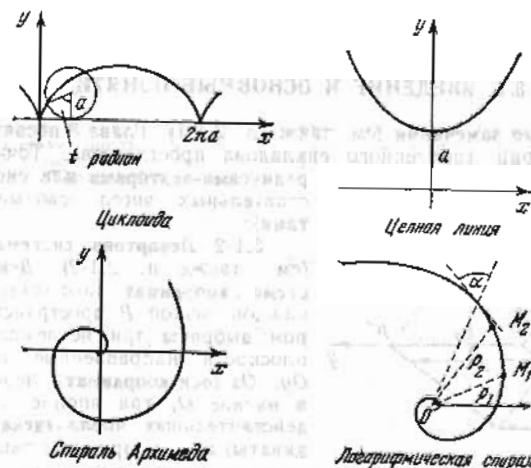
Рис. 2.6-2. Некоторые трансцендентные кривые.
