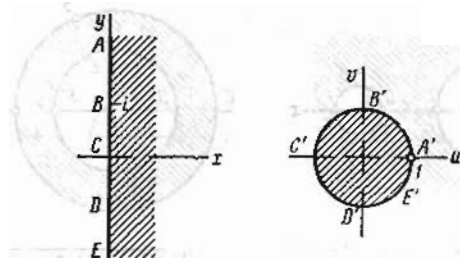
Рис. 12. w = \frac{z-1}{z+1} .
