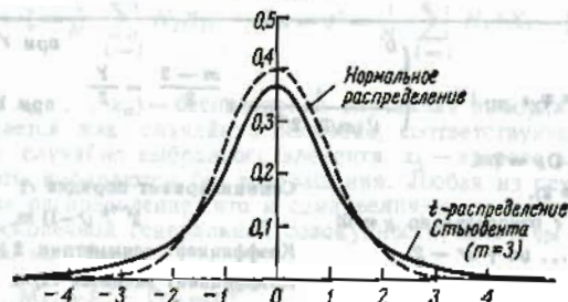
Рис. 19.5-2. t -распределение Стьюдента; сравнение со стандартизованным нормальным распределением.
