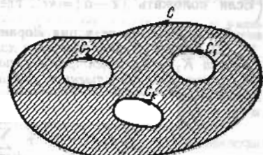
Рис. 7.5-1. Теорема Коши для много- связной области (пп. 7.2-4 и 7.5-1). Об- ласть D ограничена внешним контуром C и внутренними контурами C_1, C_2, \dots C_n ; направления обхода контуров указаны на рисунке.
