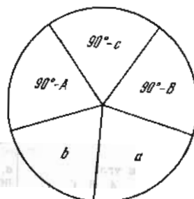
Рис. 1.12-2. Правила Непера.
