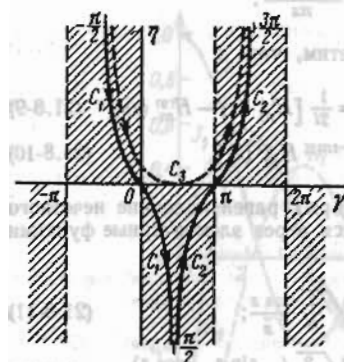
Рис. 21.8-2. Контуры интегрирования для интегралов Зоммерфельда; t = y + i\eta .
