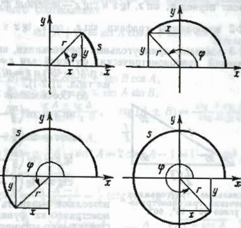
Рис. 21.2-1. Определения тригонометрических функций для данного угла \varphi .
