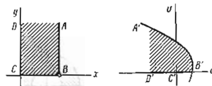
Рис. 3. w = z^2
