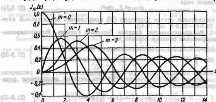
Рис. 21.8-3. Графики функций Бесселя J_0(x) , J_1(x) , J_2(x) , J_3(x) для действительного аргумента. Заметим, что J_m(-x) = (-1)^m J_m(x) .
