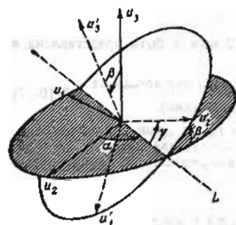
Рис. 14.10-1. Углы Эйлера \alpha, \beta, \gamma . Ось OZ второго вращения (на угол \beta ) часто называют линией узлов. Заметим, что \alpha и \beta — сферические координаты вектора u'_3 в системе u_1, u_2, u_3 .
