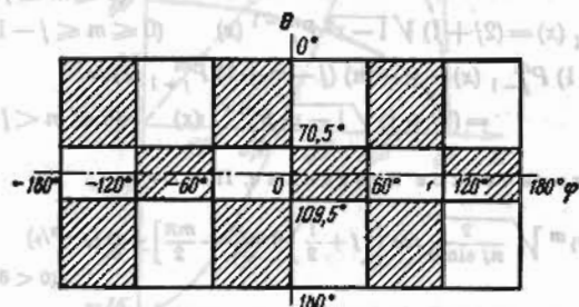
Рис. 21.8-8. Узлы функций P_j^m(\cos \theta) \sin 3\varphi на развернутой поверхности сферы. Функция отрицательная в заштрихованной части.
