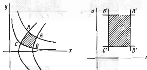
Рис. 2. w = z^2
