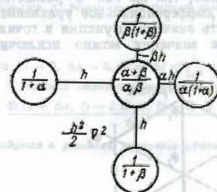
Рис. 20.9-3. Центрально-разностный оператор, применяемый для градуированной сетки или для аппроксимации вблизи границы. Относительная погрешность имеет порядок h .
