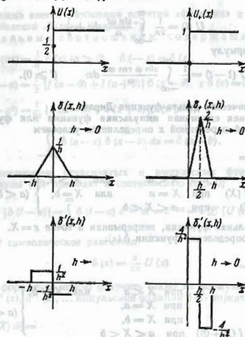
Рис. 21.9-1. Единичные ступенчатые функции U(x) и U_+(x) и аппроксимация импульсных функций \delta(x) , \delta_+(x) , \delta'(x) и \delta'_+(x) .
