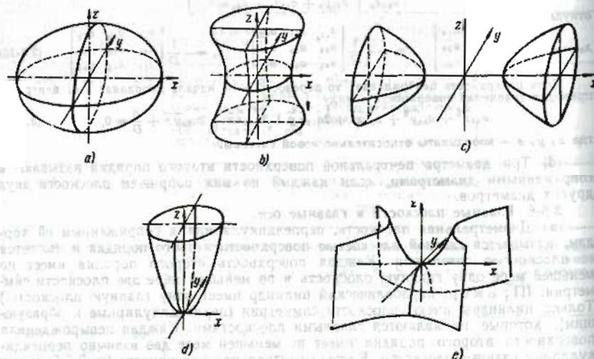
Рис. 3.5-1. Невырожденные поверхности второго порядка: а) эллипсоид, б) однополостный гиперболоид, в) двуполостный гиперболоид, г) эллиптический параболоид, д) гиперболический параболоид.
