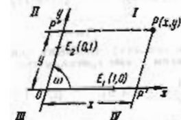
Рис. 2.1-1. Правая декартова координатная система координат. Отрезки OP' и OP'' — единицы масштаба на осях
